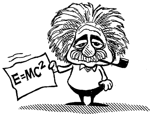
EINSTEIN'S
