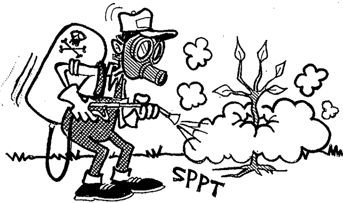
HERBICIDE
