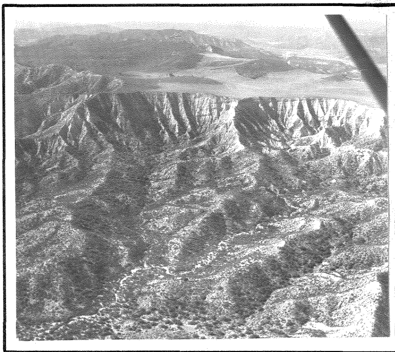
Figure 10 - Scalloped edge of Puckett Mesa.
